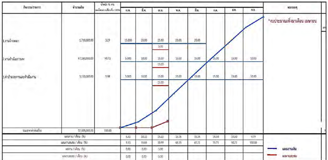
แผน - ผลปฏิบัติงานก่อสร้าง โครงการก่อสร้าง เขื่อนกั้นคลองชลประทานที่ 1 งานเสริมสันเขื่อนเพิ่มความจุอ่างเก็บน้ำอ่างเก็บน้ำแม่ปอน อันเนื่องมาจากพระราชดำริ ตำบลแม่หอพระ อำเภอแม่แตง จังหวัดเชียงใหม่ ประจำปีคชชน เมษายน 2560
